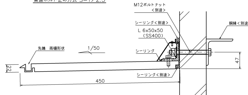
貫通ボルト止め方式 S=1/2.5
