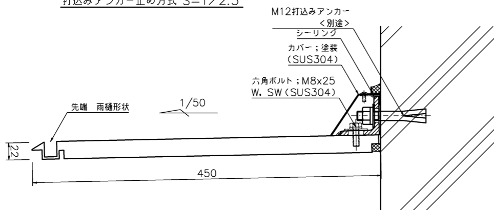
打込みアンカー止め方式 S=1/2.5
