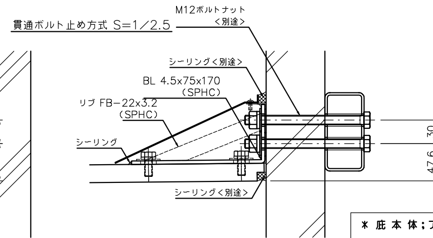
側面部材拡大図 S=1/2.5
