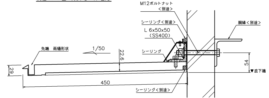
貫通ボルト止め方式 S=1/2.5
