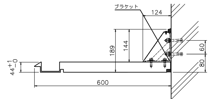
貫通ボルト止め方式 S=1/2.5
