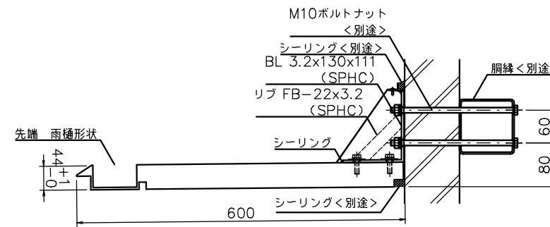
貫通ボルト止め方式 S=1/5
