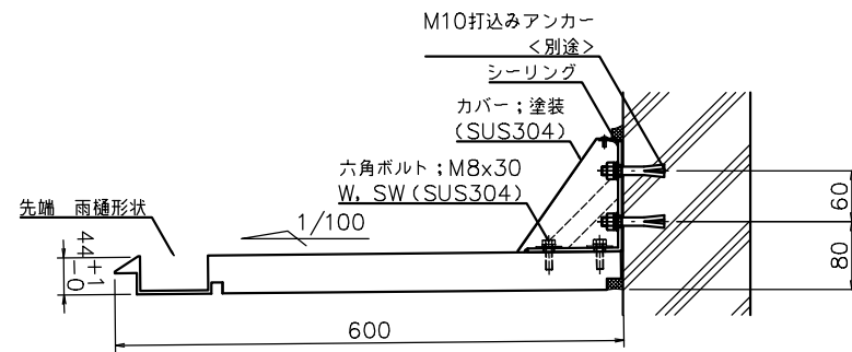
打込みアンカー止め方式 S=1/5
