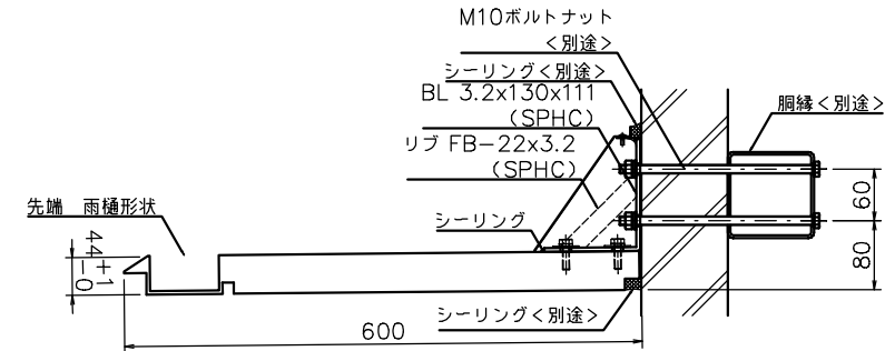
貫通ボルト止め方式 S=1/5
