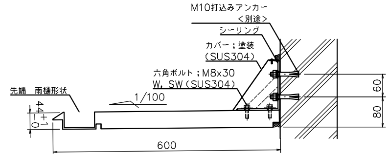
打込みアンカー止め方式 S=1/5
