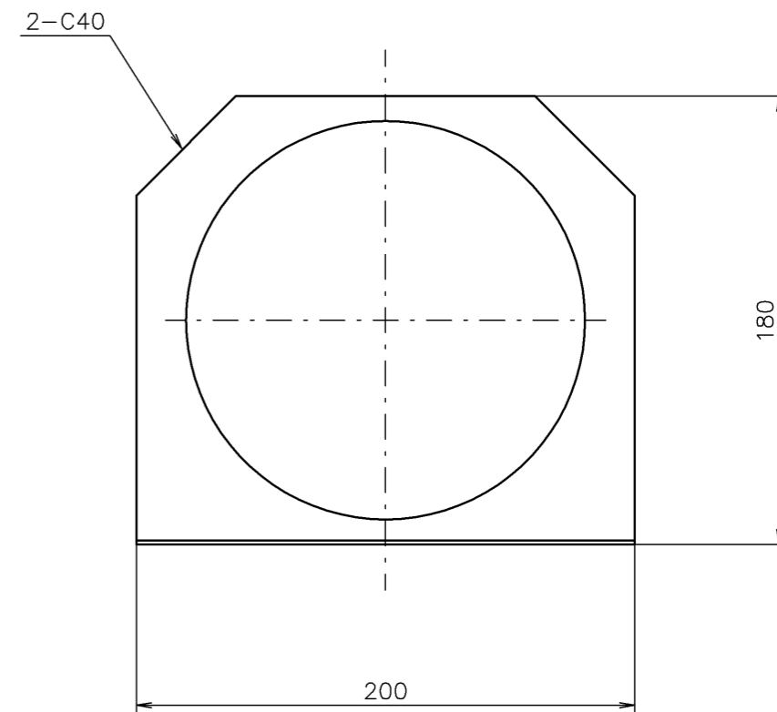
A矢視図
