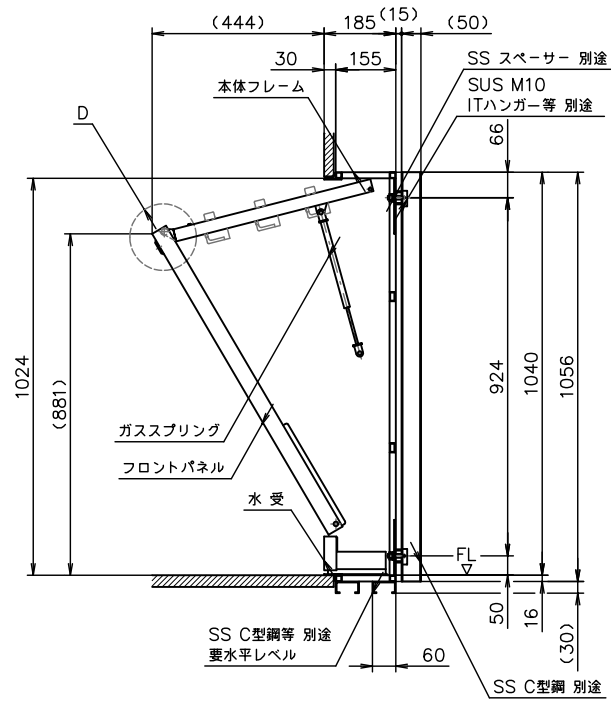
PIR-B11-1309H 外観図 S=1:10 傘収納本数：27本
