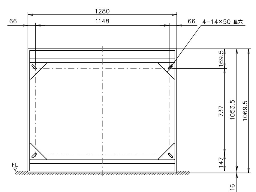
本体フレーム背面 壁面取付穴位置図 S=1:10
