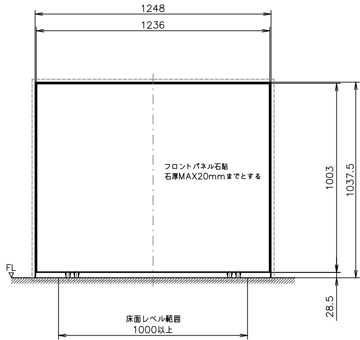
PIR-C11-1312H 外観図 S=1:10
