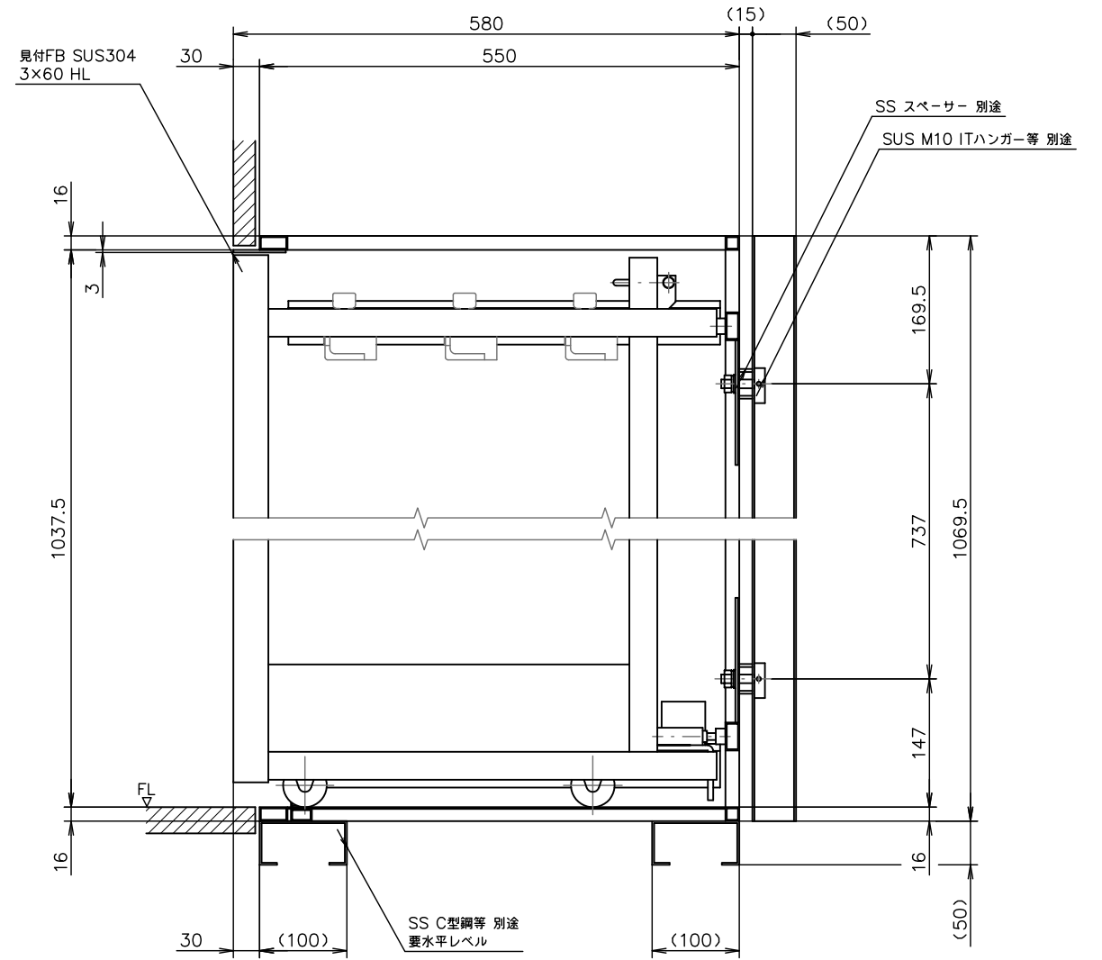
B・C部詳細図 S=1:4
