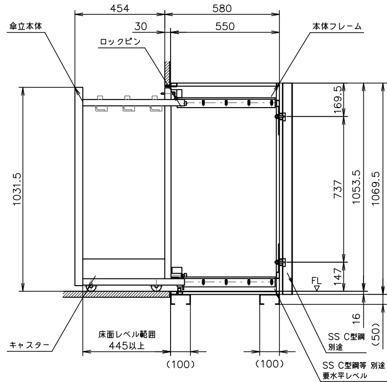
PIR-C11-1312H 外観図 S=1:10
