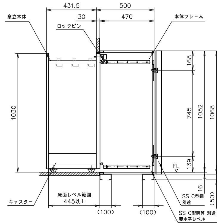
PIR-C12-1309H 外観図 S=1:10 傘収納本数: 30本
