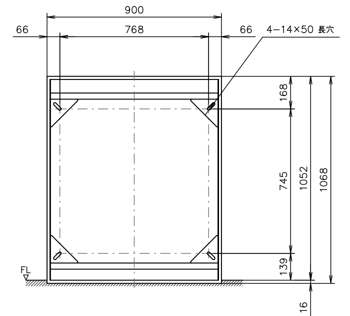
本体フレーム背面 壁面取付穴位置図 S=1:10
