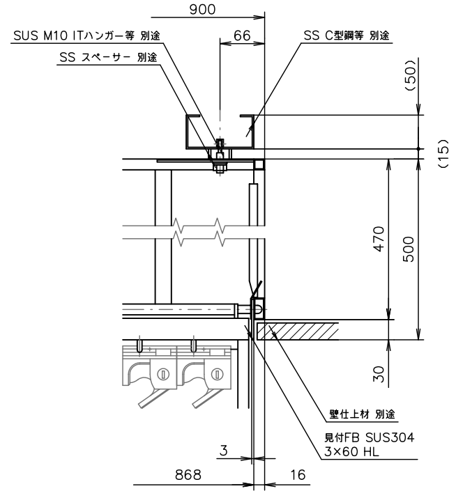
A部詳細図 S=1:4
