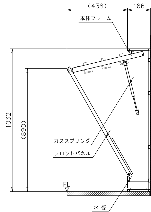
PIR-D12-1309 外観図 S=1:10
