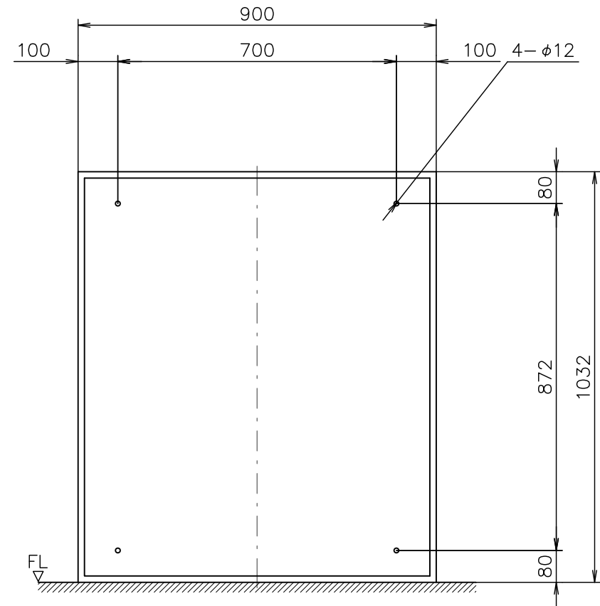
本体フレーム背面 壁面取付穴位置図 S=1:10
