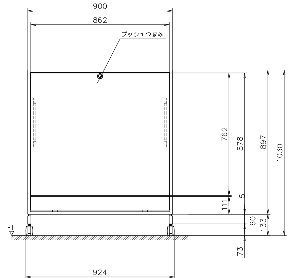
PIR-D1S-1309H 外観図 S=1:10 傘収納本数：27本
