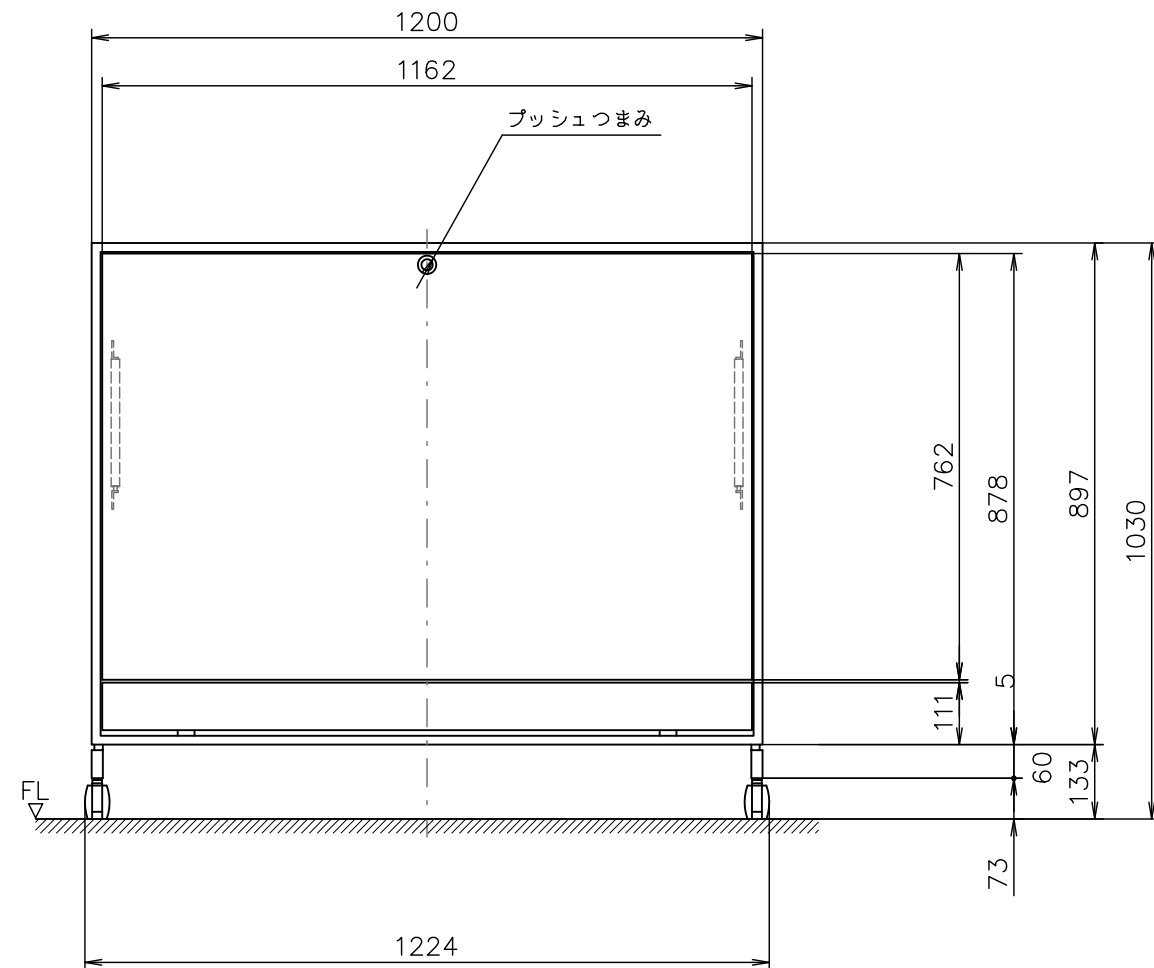
PIR-D1S-1312H 外観図 S=1:10
