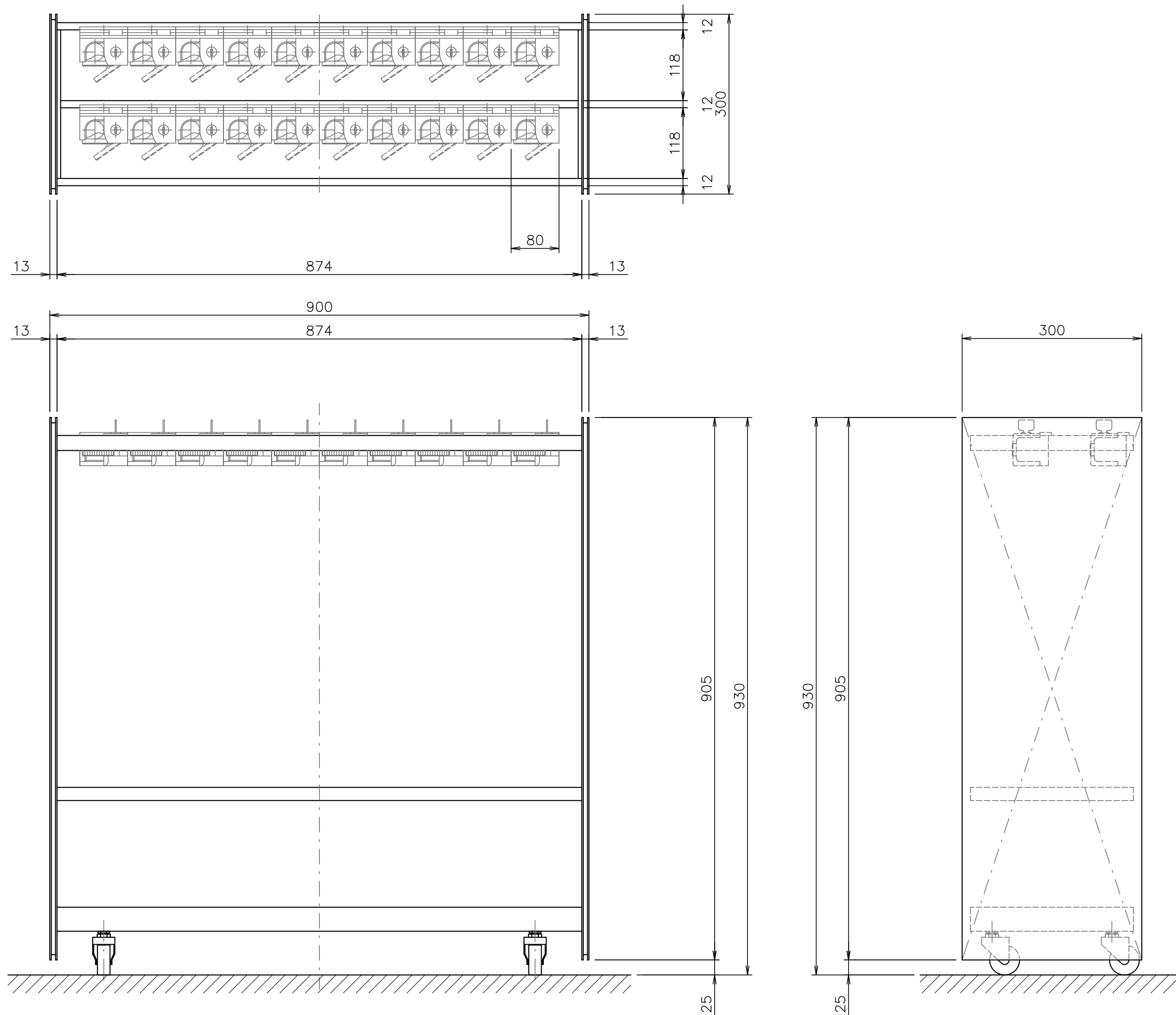
PIR-H12-1209H 外觀図 S=1:5
