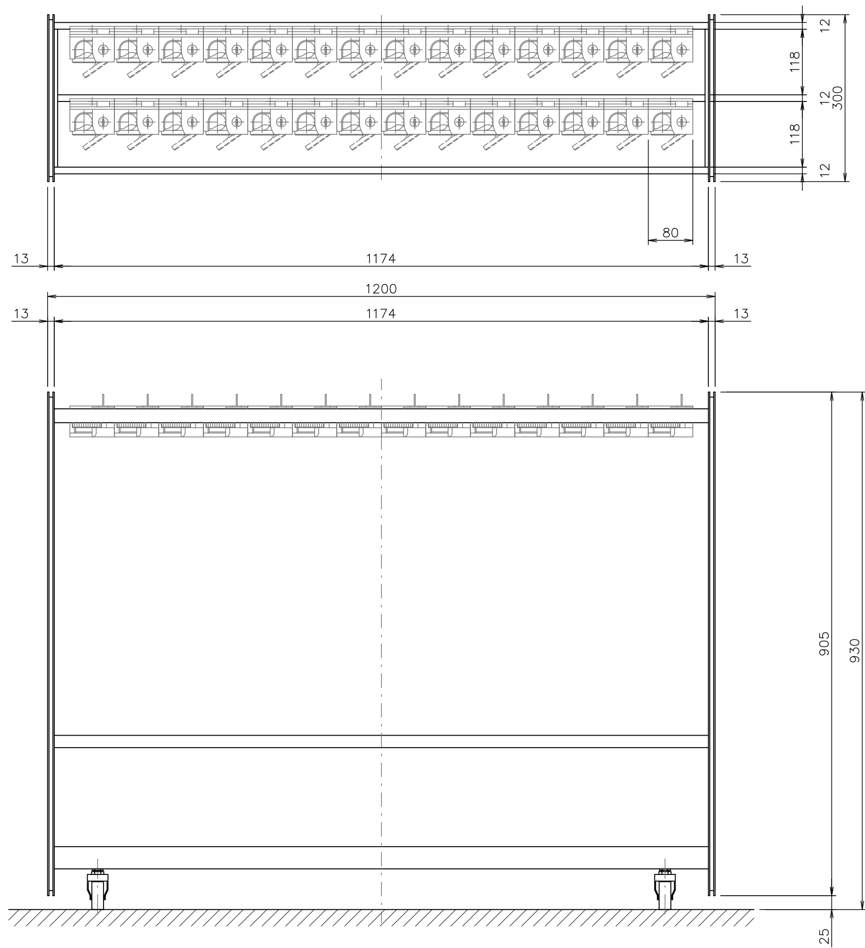
PIR-H12-1212H 外觀図 S=1:5
