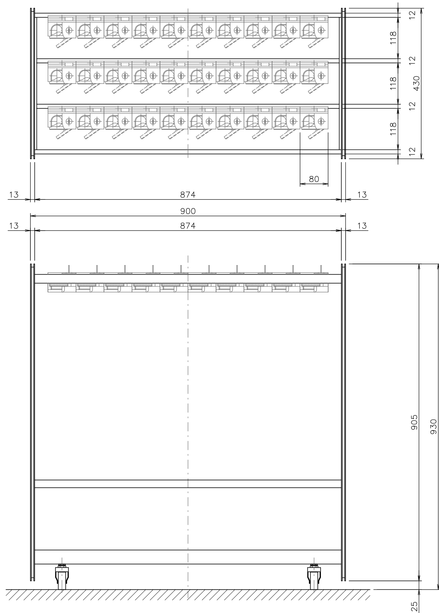
PIR-H12-1309H 外觀図 S=1:5
