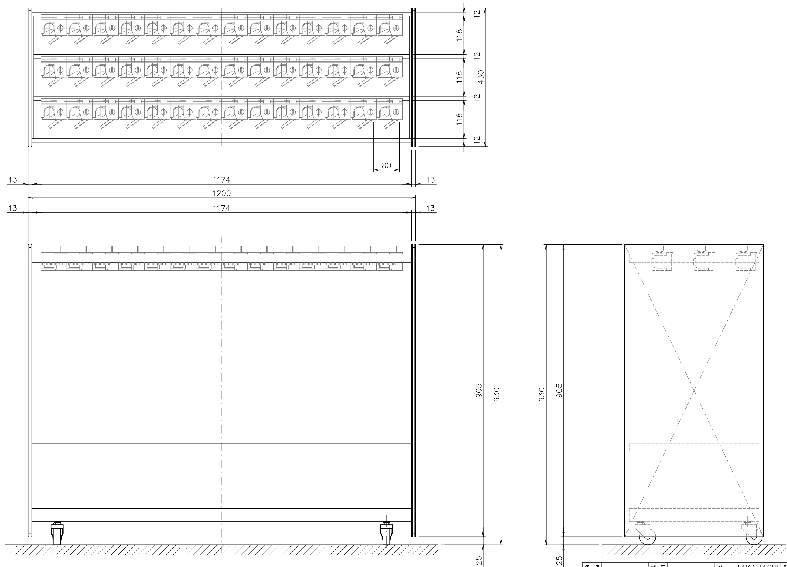
PIR-H12-1312H 外觀図 S=1:5
