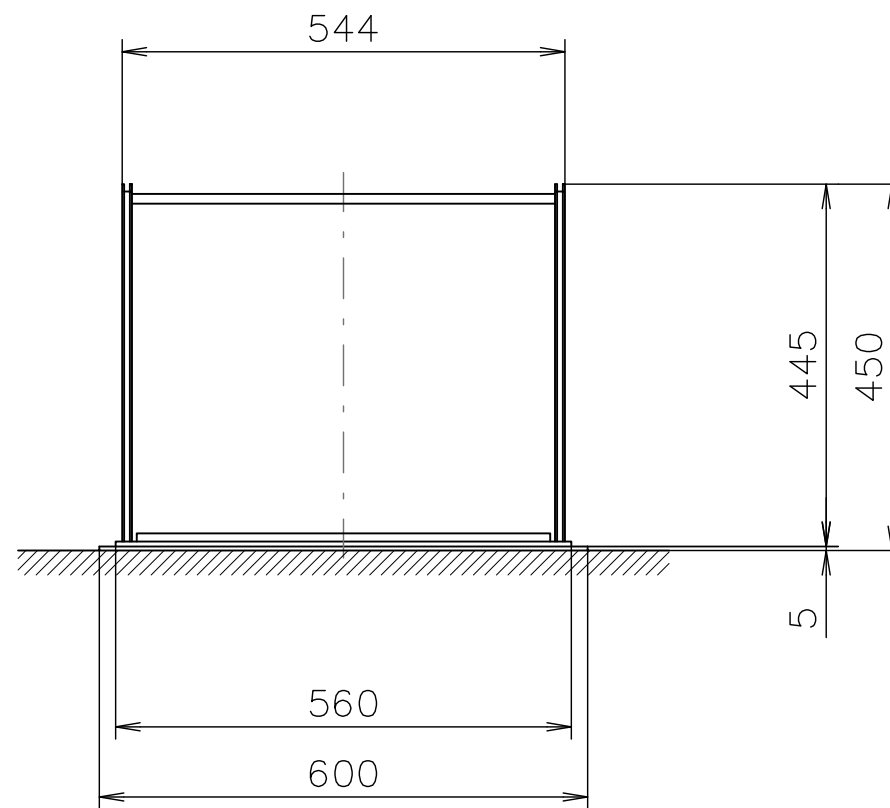
PIR-H22-2106H-AL-S 外觀図 S=1:10
