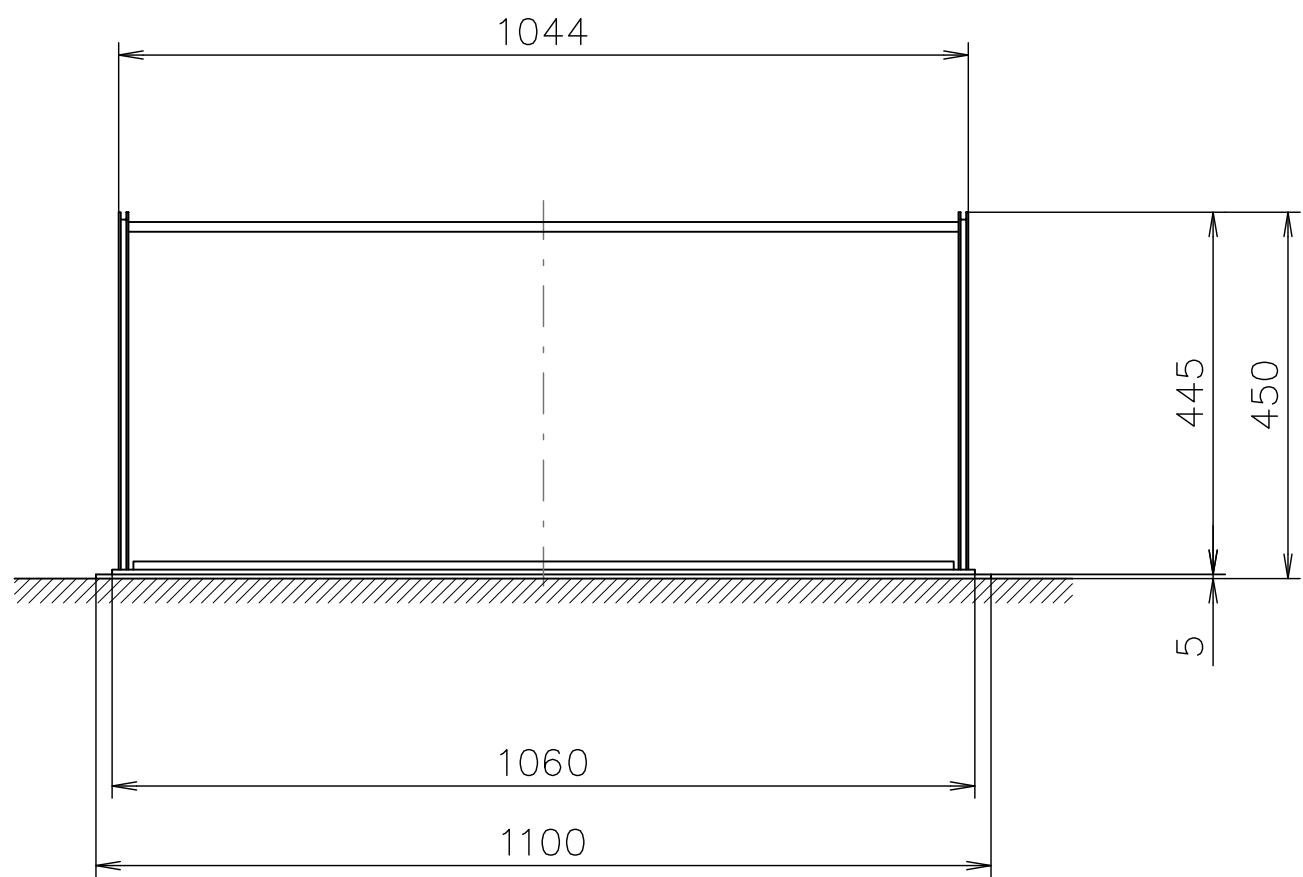
PIR-H22-2110H-AL-S 外觀図 S=1:10
