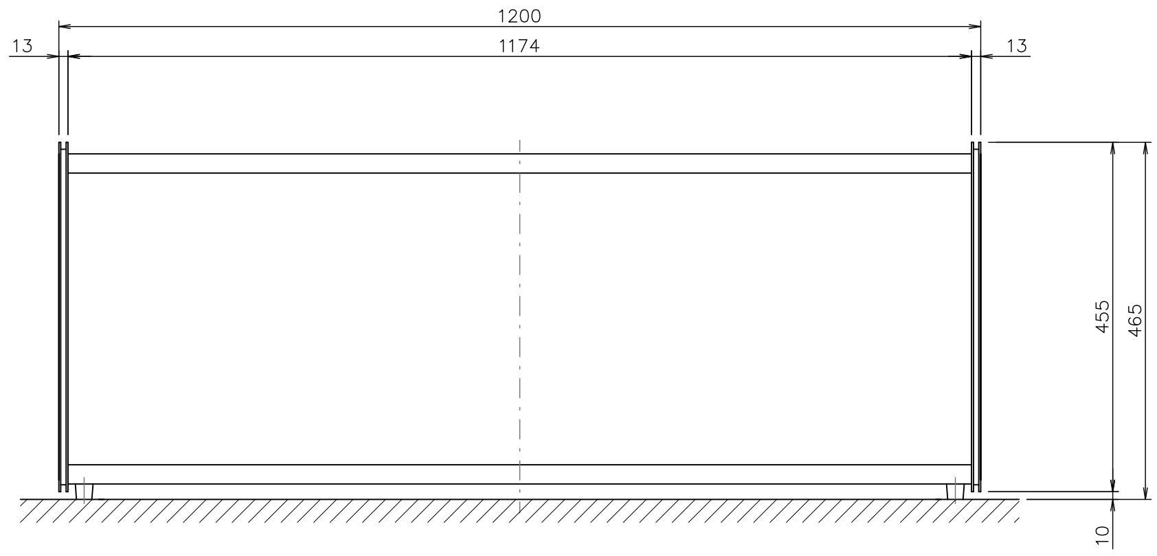
PIR-H22-2212H-AL 外観図 S=1:5 傘収納本数：24コマ 24~48本
