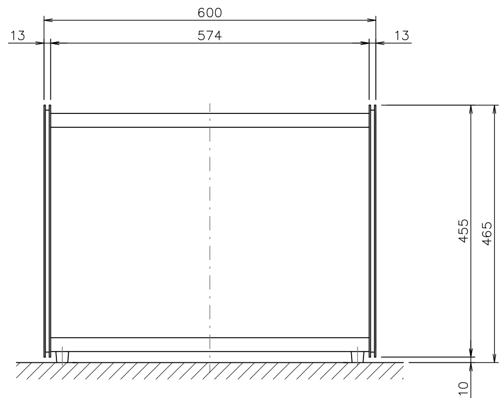
PIR-H22-2306H-AL 外觀図 S=1:5 傘収納本数: 18コマ 18~36本
