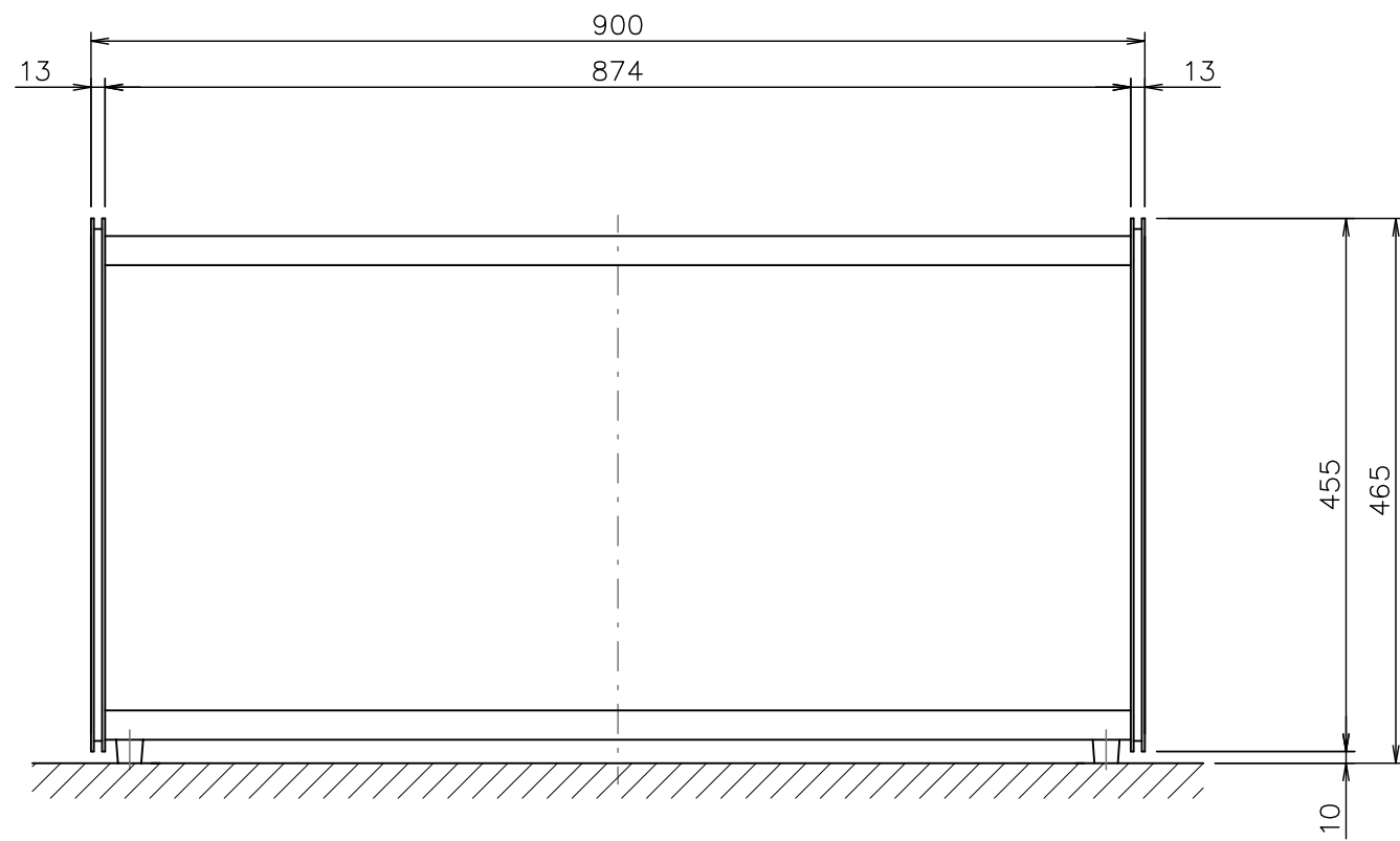
PIR-H22-2309H-AL 外觀図 S=1:5 傘収納本数：27コマ 27~54本
