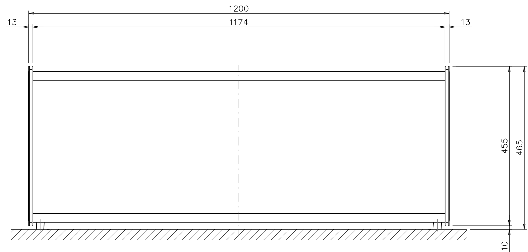
PIR-H22-2312H-AL 外觀図 S=1:5 傘収納本数：36コマ 36~72本
