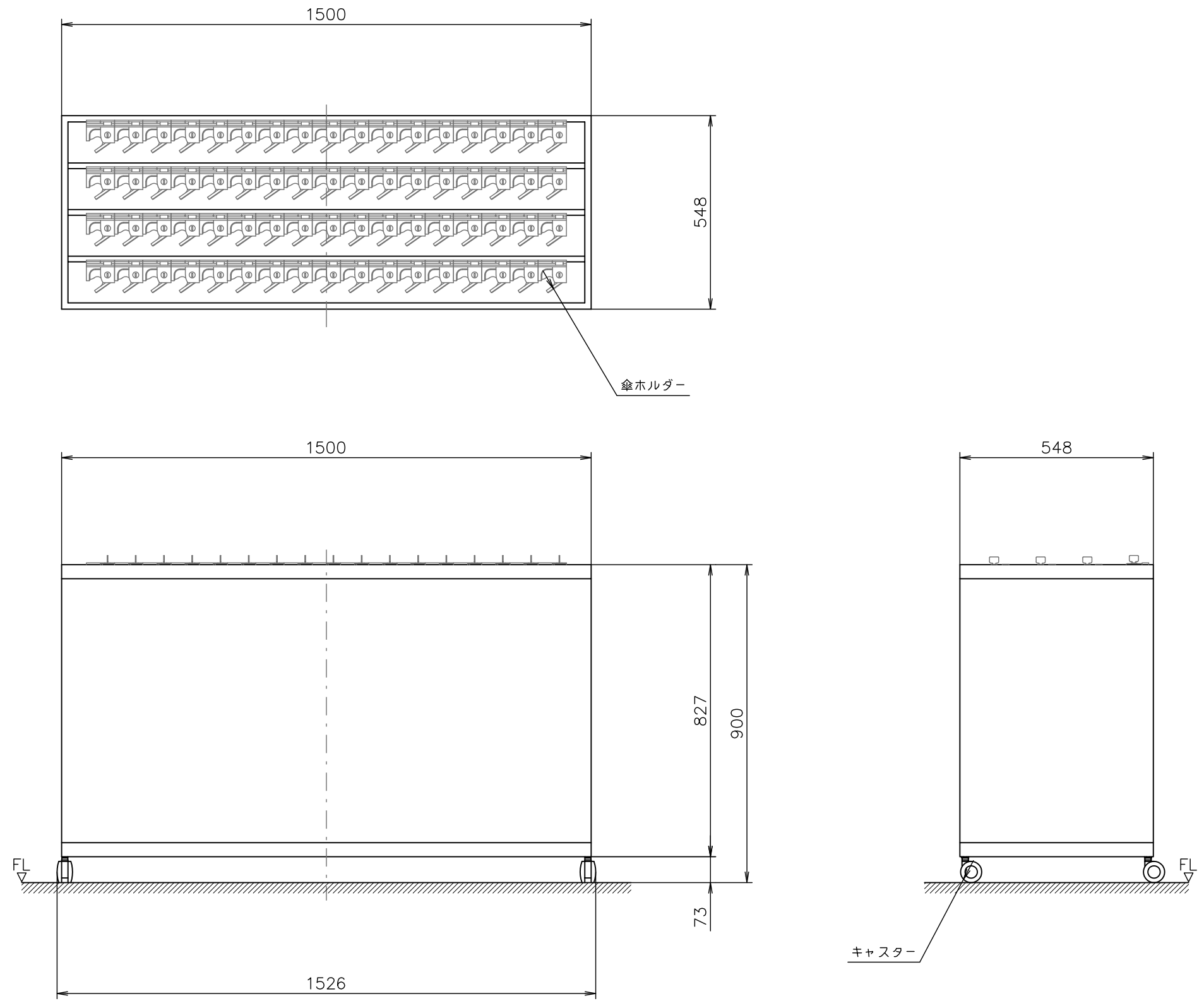
PIR-M12-1415H 外観図 S=1:10 傘収納本数：68本
